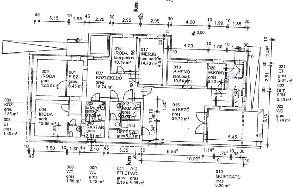
átalakítás, bővítés alaprajza
