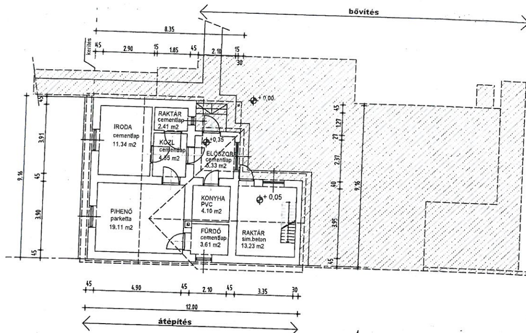
jelenlegi állapot alaprajza
